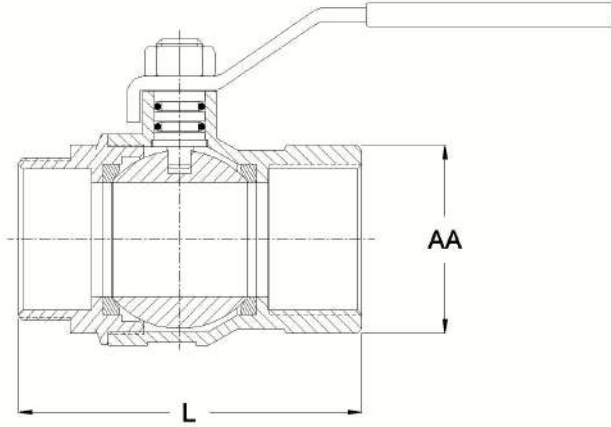
PN25 Erkek x Dişi Küresel Vana Ölçü Tablosu
