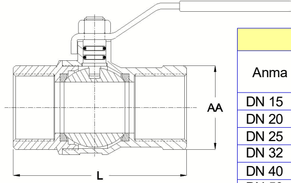
Küresel Kosva Vana Ölçü Tablosu
