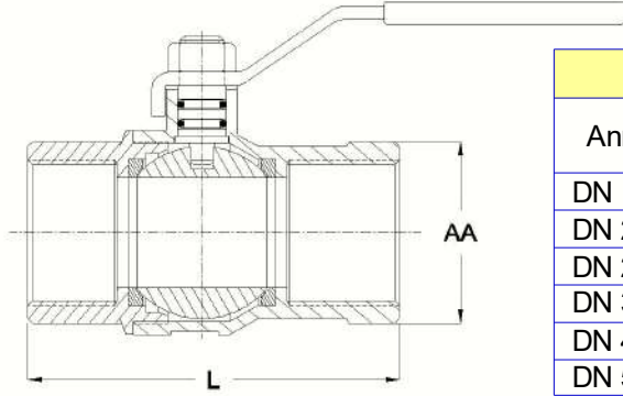
PN16 Küresel Vanalar Ölçü Tablosu
